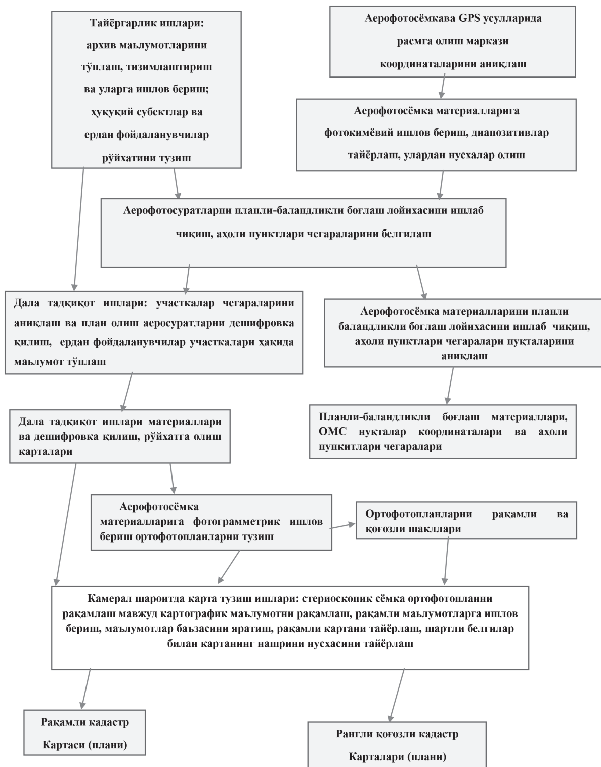
1-блок схема
